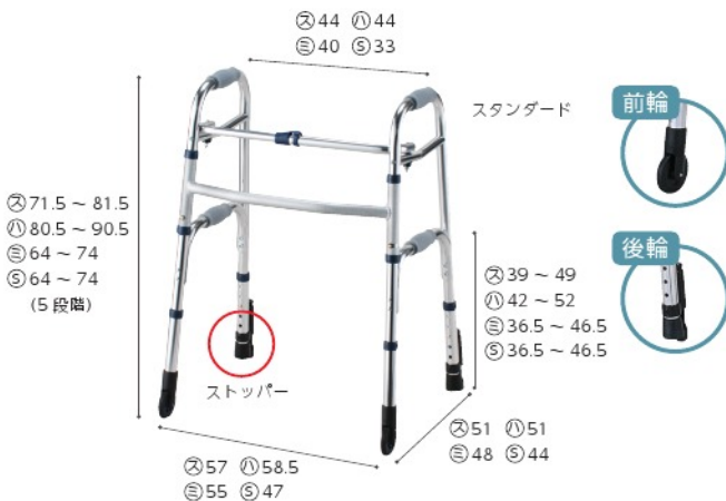
単位：cm ㉔：スタンダード ㉕：ハイタイプ ㉖：ミニ ㉗：SS
