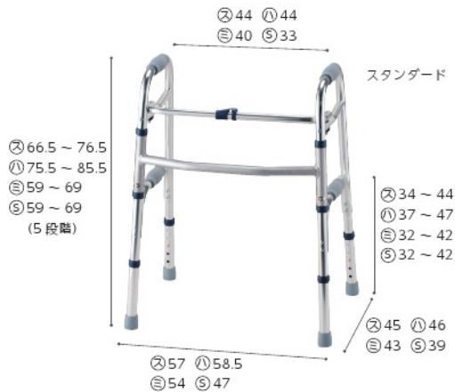
単位：cm ㉔：スタンダード ㉕：ハイタイプ ㉖：ミニ ㉗：SS
